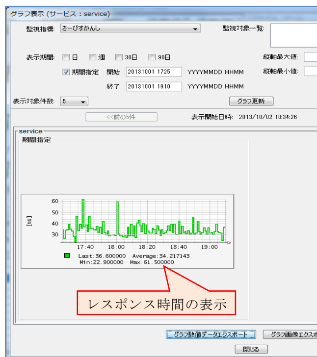
図 3 : レスポンス時間表示画面
