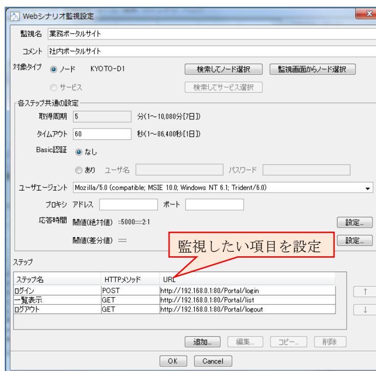
図 2 : Web シナリオ監視設定画面
